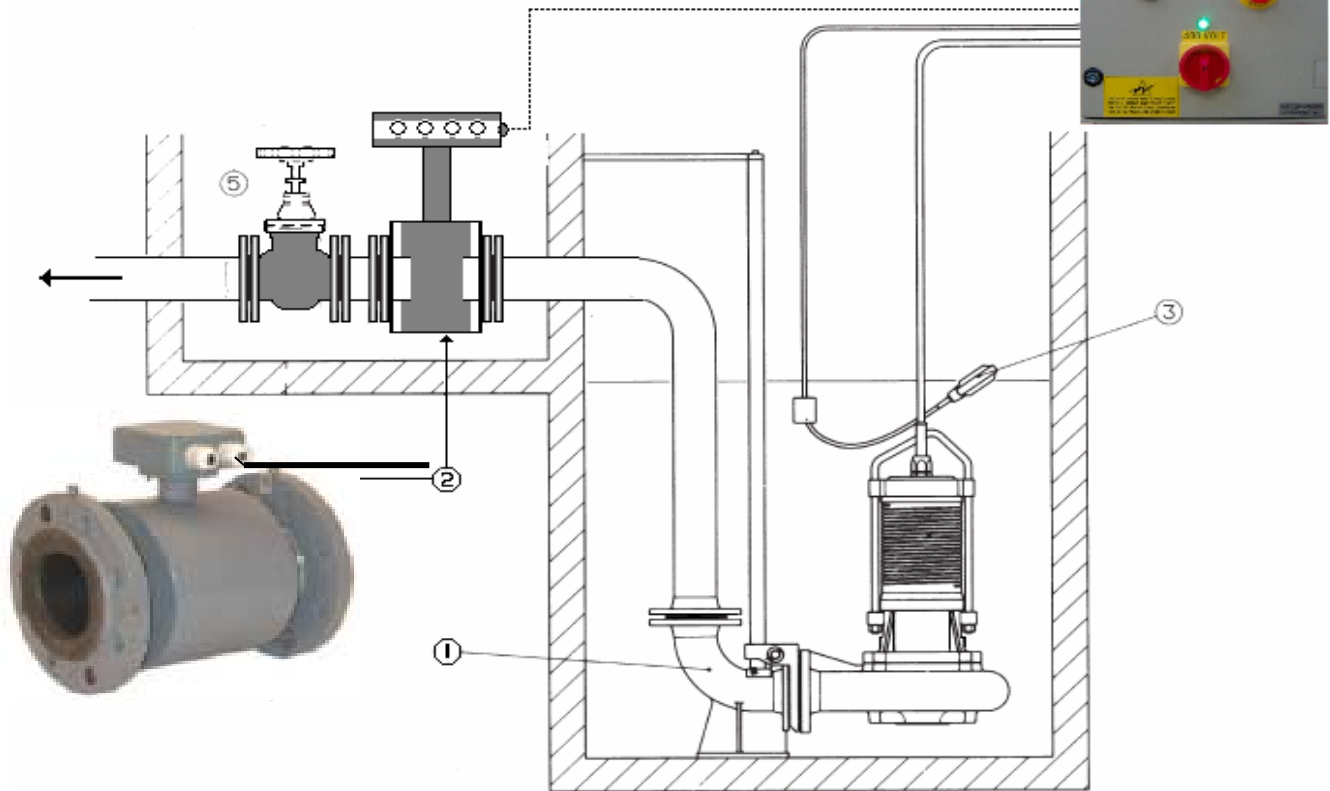
SVOTAMENTO AUTOMATICO DEL POZZETTO CON REGISTRAZIONE LOCALE E REMOTA DEI LITRI EVACUATI CONTABILIZZAZIONE DIRETTA SU PC
